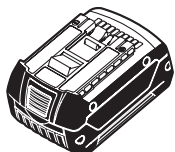
18 V (Li-Ion) 2 607 336 170 (1,3 Ah „compact“) 2 607 336 092 (2,6 Ah) 2 607 336 236 (3,0 Ah)
