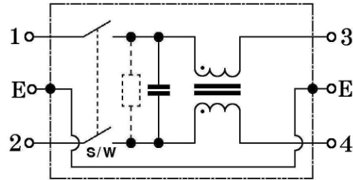
RIR3-***0 TYPE
