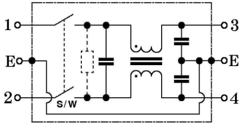
RIR3-**** TYPE
