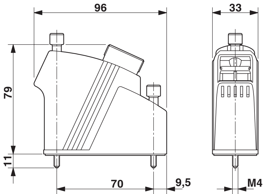
尺寸图
