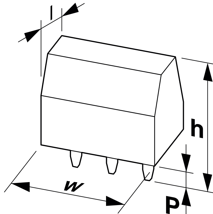
尺寸图
