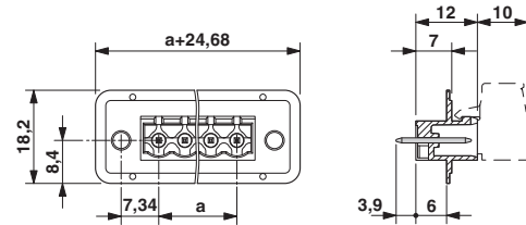
外形寸法
