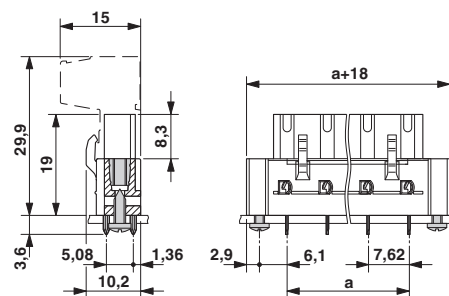
外形寸法
