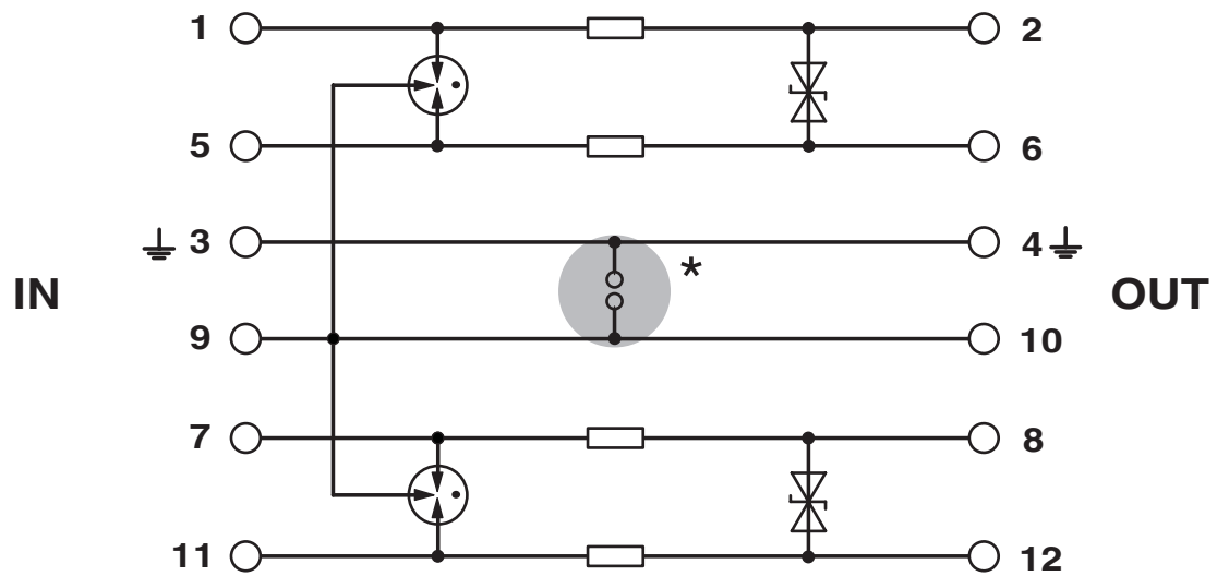
电路图
