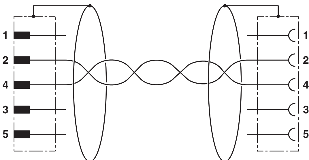
电路图
