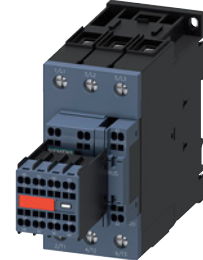
3RT203.-3NB34-3MA0
