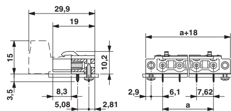
外形寸法
