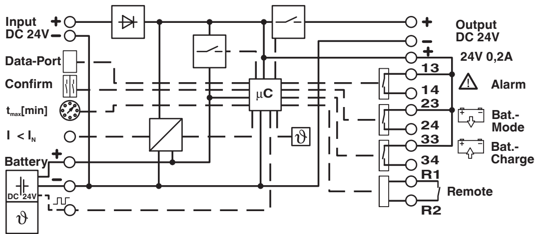
Blockschaltbild
