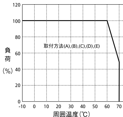
強制空冷時の 出力ディレーティング (標準品及びL板金付)
