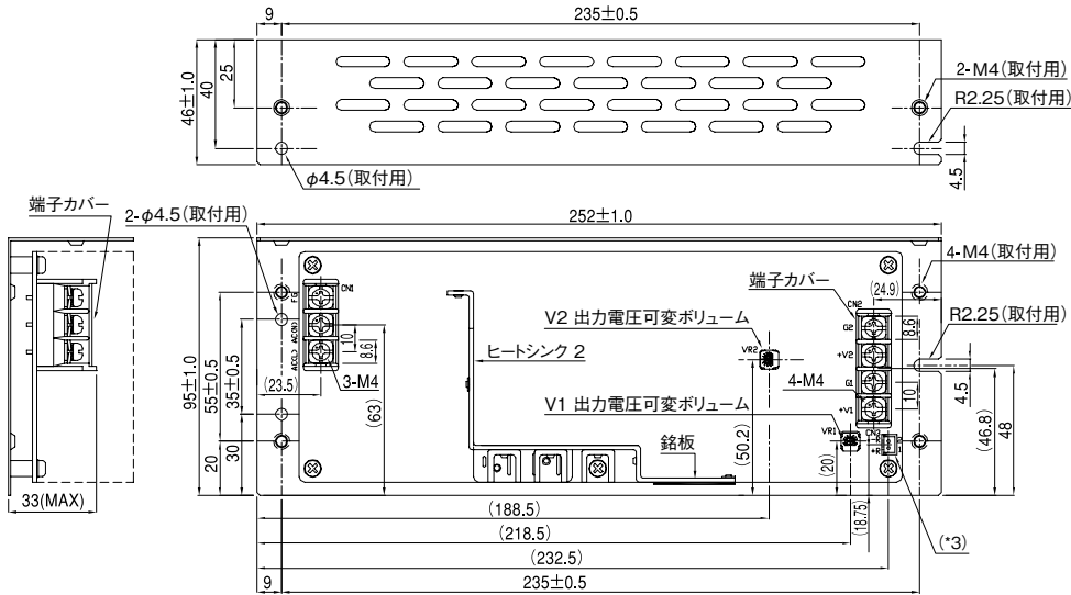
[ZWD150PAF (TL仕様：端子台垂直方向, L板金タイプ)]
