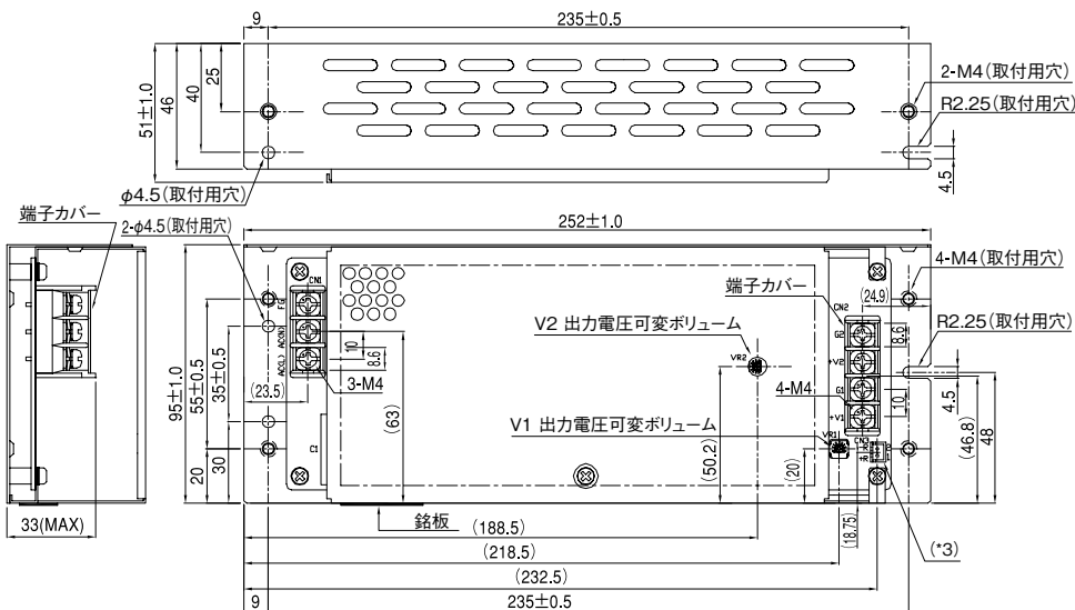
[ZWD150PAF (TA仕様：端子台垂直方向, カバー付タイプ)]
