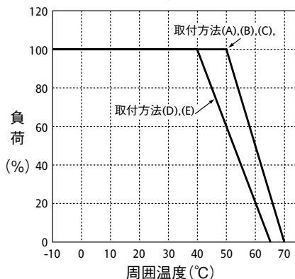
自然空冷時の 出力ディレーティング (標準品及びL板金付)
