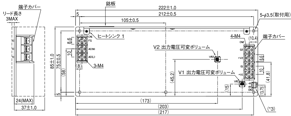
[ZWD150PAF (T仕様：端子台垂直方向タイプ)]
