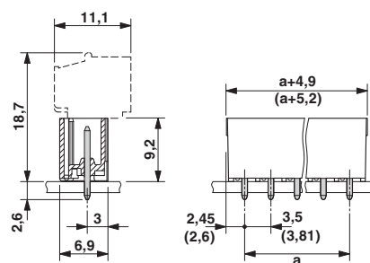
外形寸法
