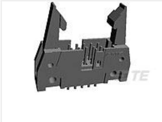
TE Part #5499374-8 A/L UNIV HDR 34P VERT SHT LAT
