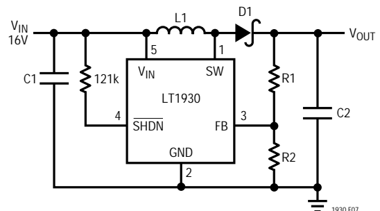
図7 . 10V以下に保たれたSHDN
