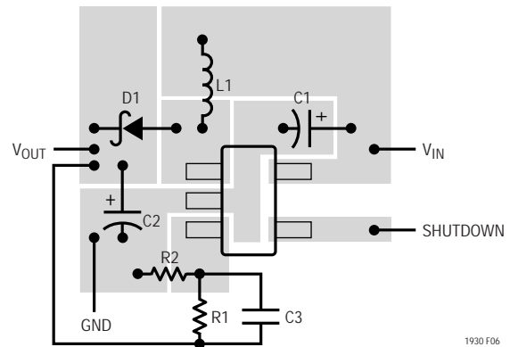
図6 . 推奨レイアウト
