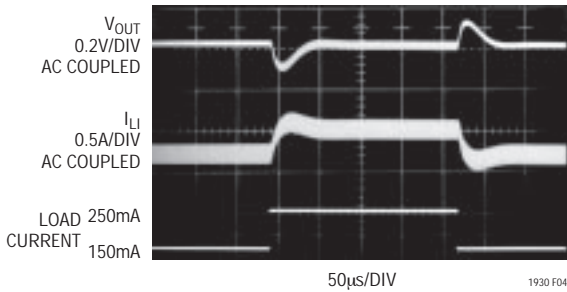
図4 . 10pFの位相リード・コンデンサを使った昇圧コンバータの過渡応答
