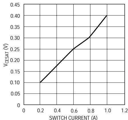
スイッチ飽和電圧
