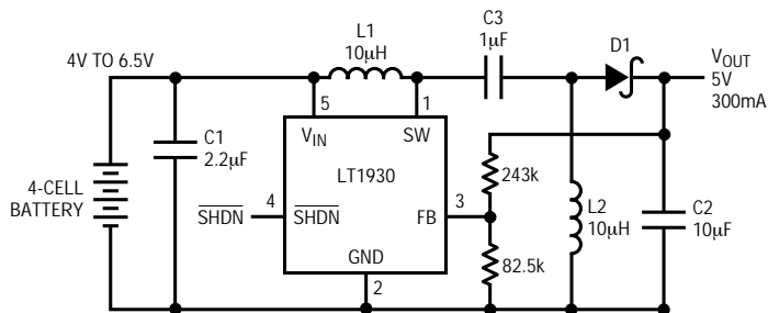
4セル動作の5V SEPICコンバータ
