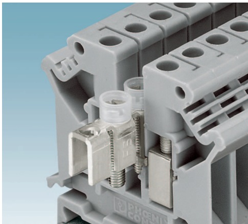
Bild 11 Feste Brücke
