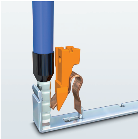
Bild 3 Push-in-Anschluss
