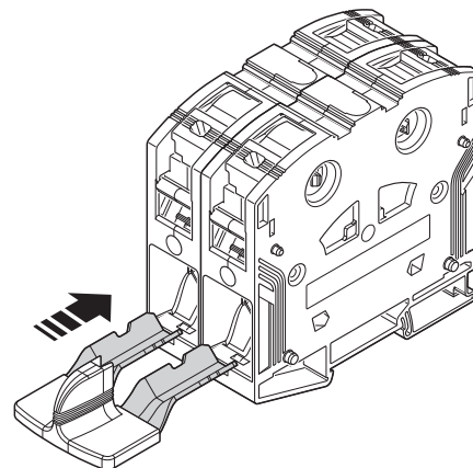
Bild 9 Einlegebrücken
