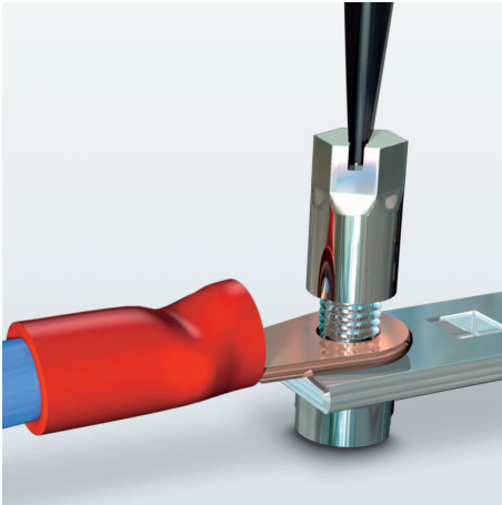
Bild 5 Bolzenanschluss
