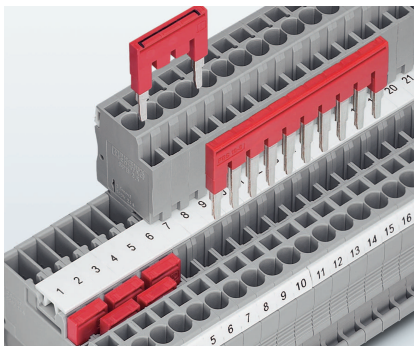
Bild 8 Steckbrücken
