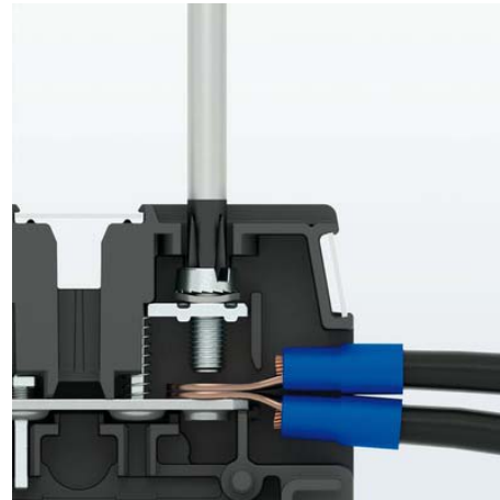
Bild 6 Barrier-Anschluss
