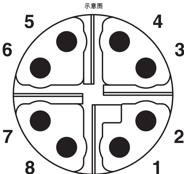
M12连接器, Cat6 A , 8芯, 引脚分配, 插头侧视图
