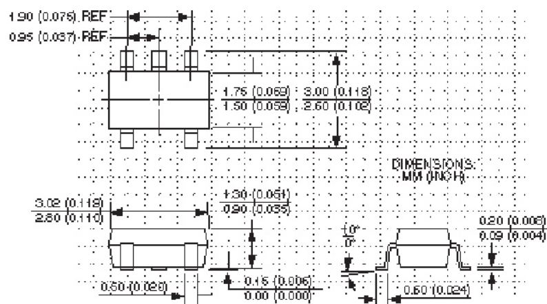
SOT-23-5 (M5)
