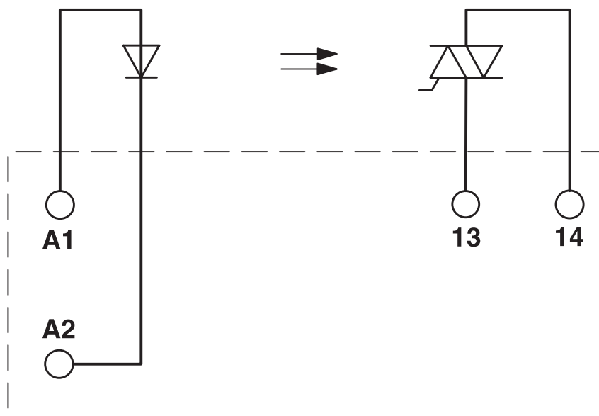
电路图
