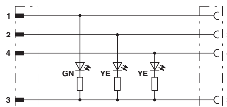
回路図
