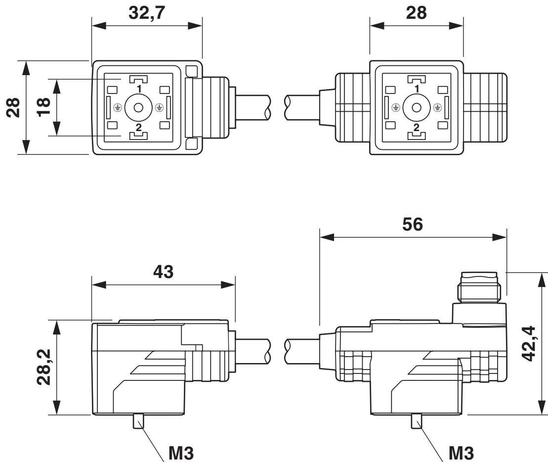
尺寸图
