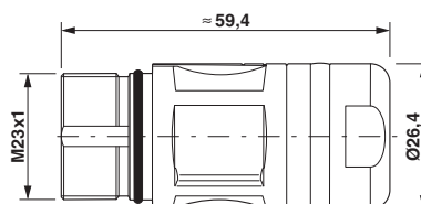
外形寸法
