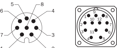
电缆/外壳上的设备插头 M12 / M23 视图
