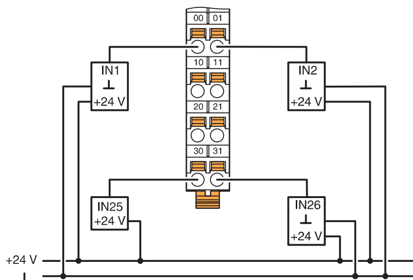
接线图
