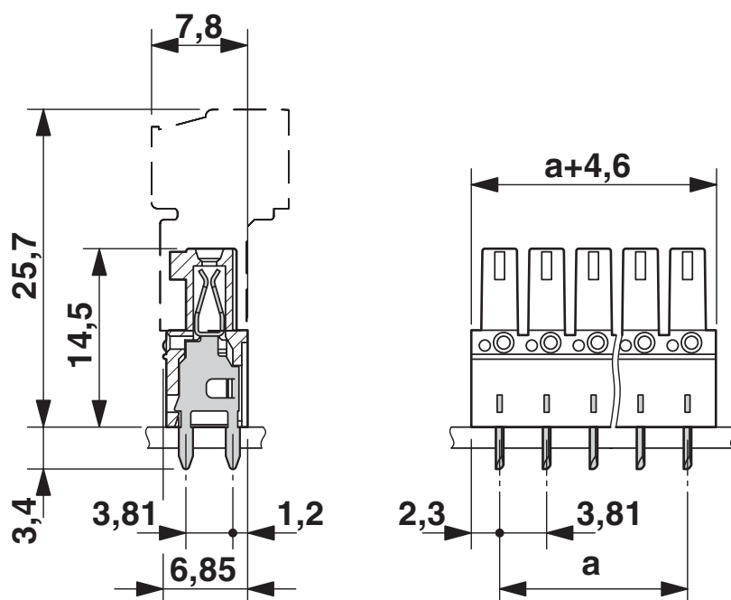
尺寸图
