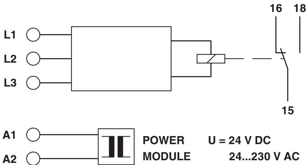
Blockschaltbild
