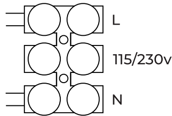
Diagrama eléctrico 2 (CA)
