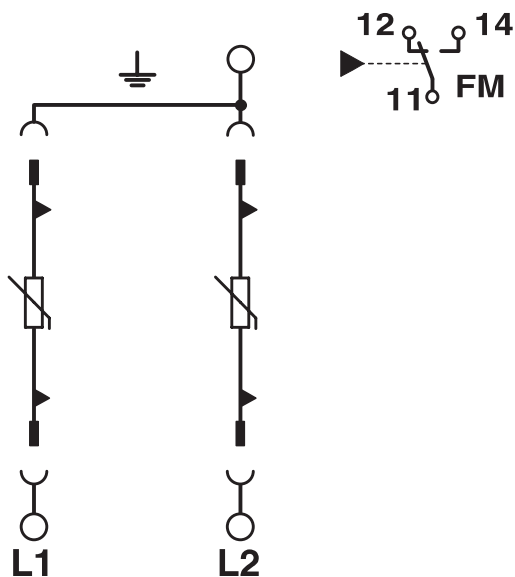
电路图
