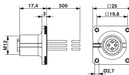
外形寸法
