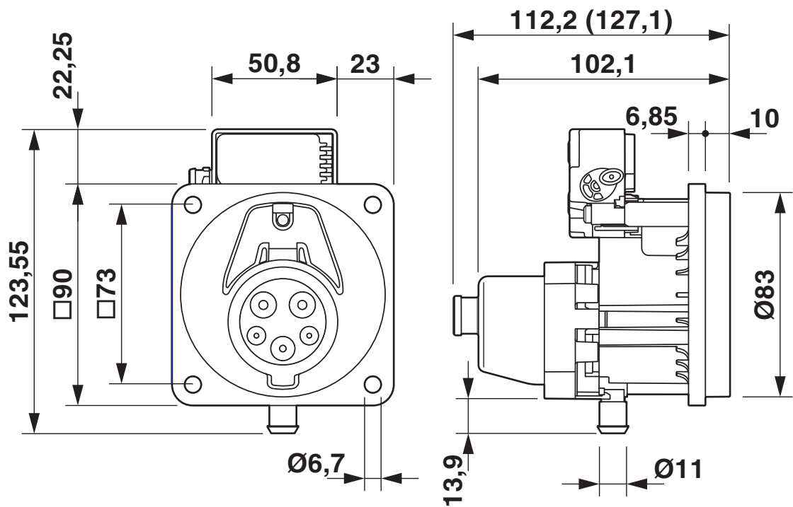
尺寸图
