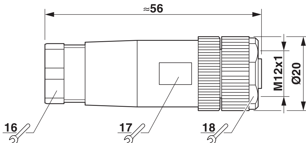
尺寸图
