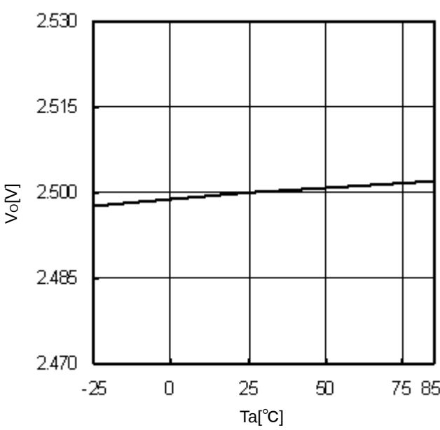
Fig.10 T_a-V_o (I_o=0A)
