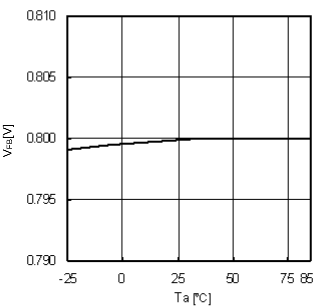
Fig.9 T_a-V_{FB}
