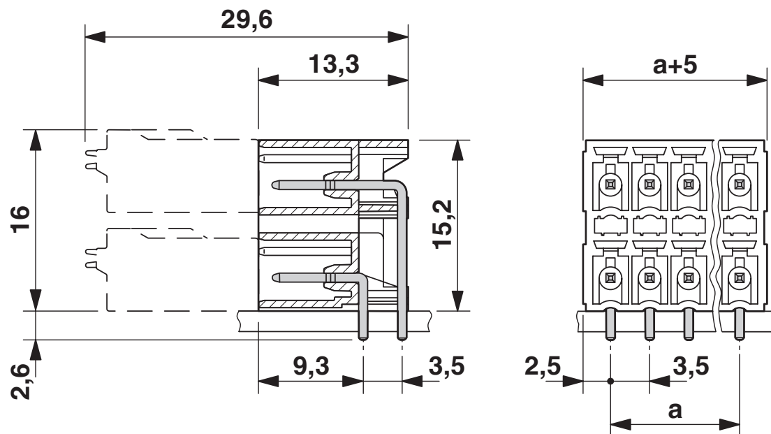
尺寸图
