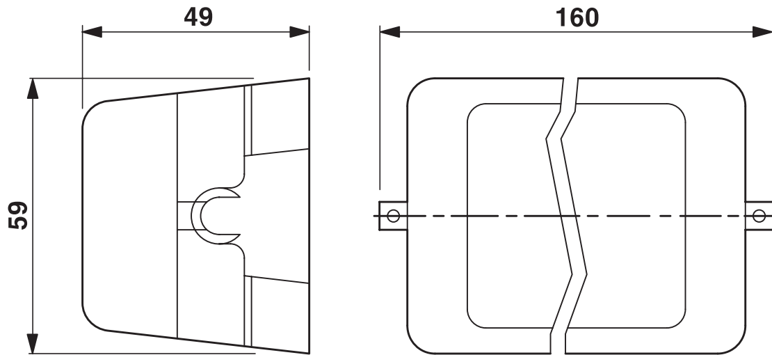
尺寸图
