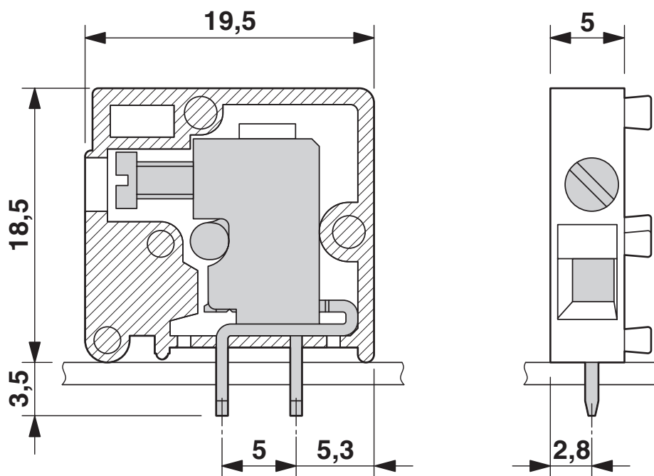
尺寸图
