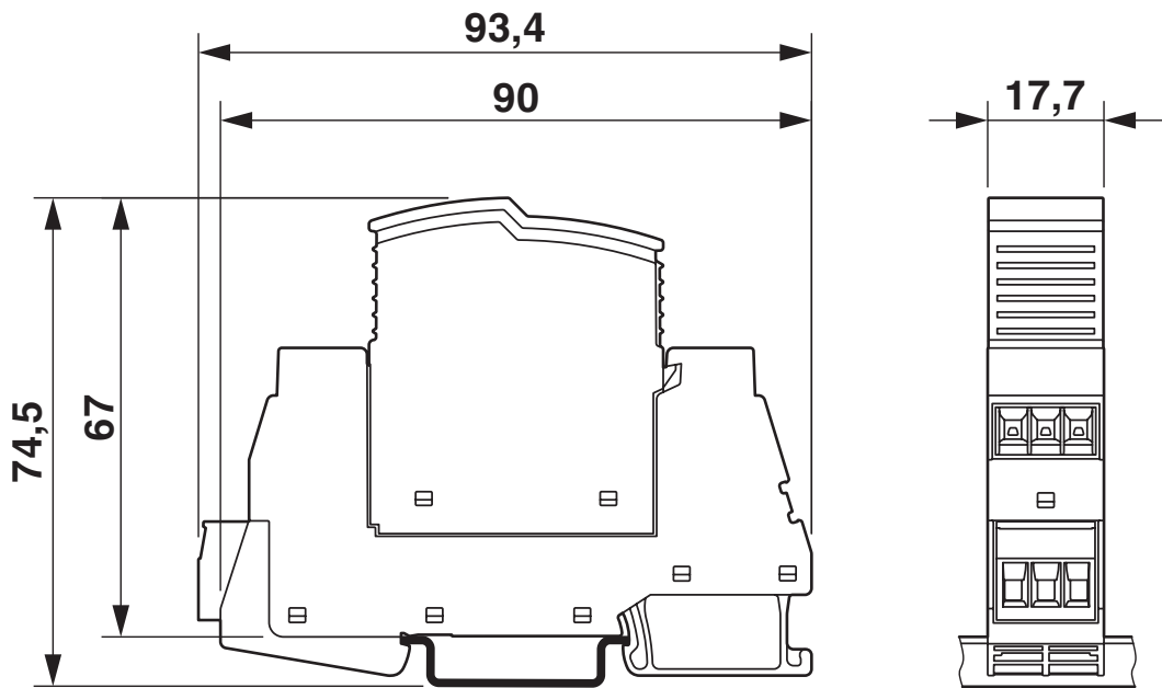
尺寸图
