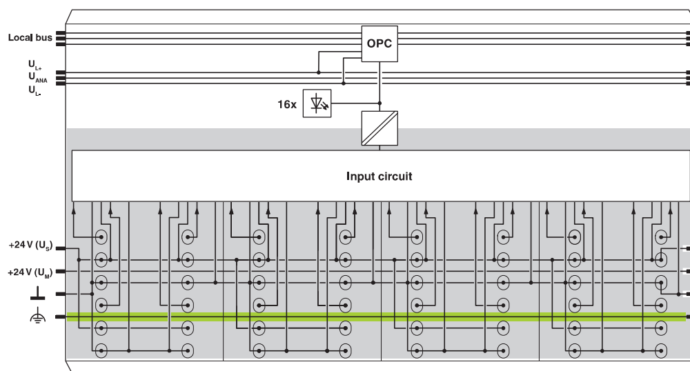
结构框图
