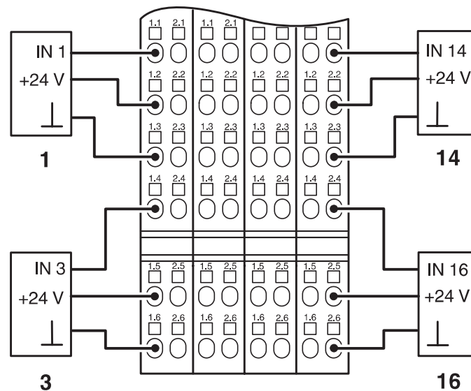
接线图
