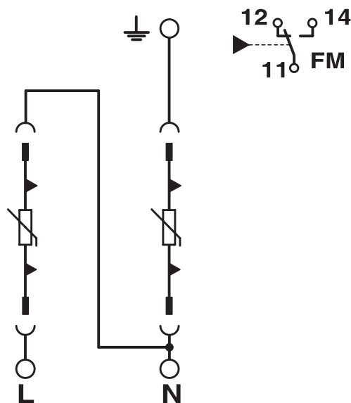
电路图
