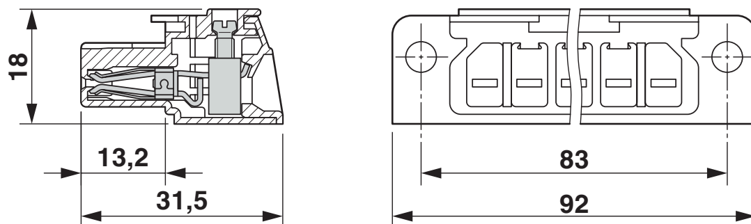
尺寸图
