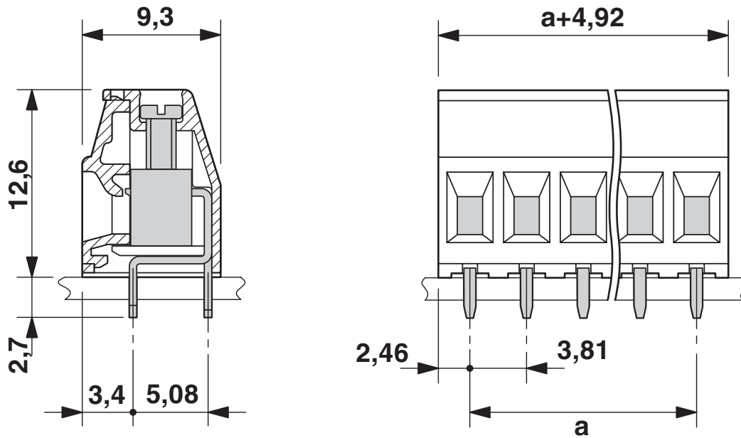
尺寸图
