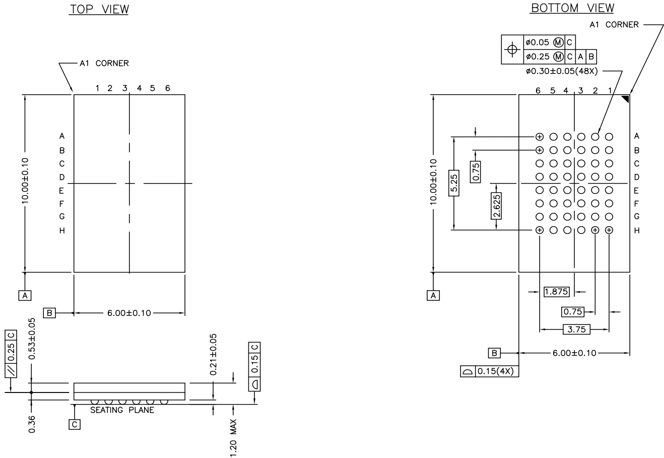
図 19. 48 ボール FBGA ( 6 × 10 × 1.2mm ) パッケージ図、51-85128
