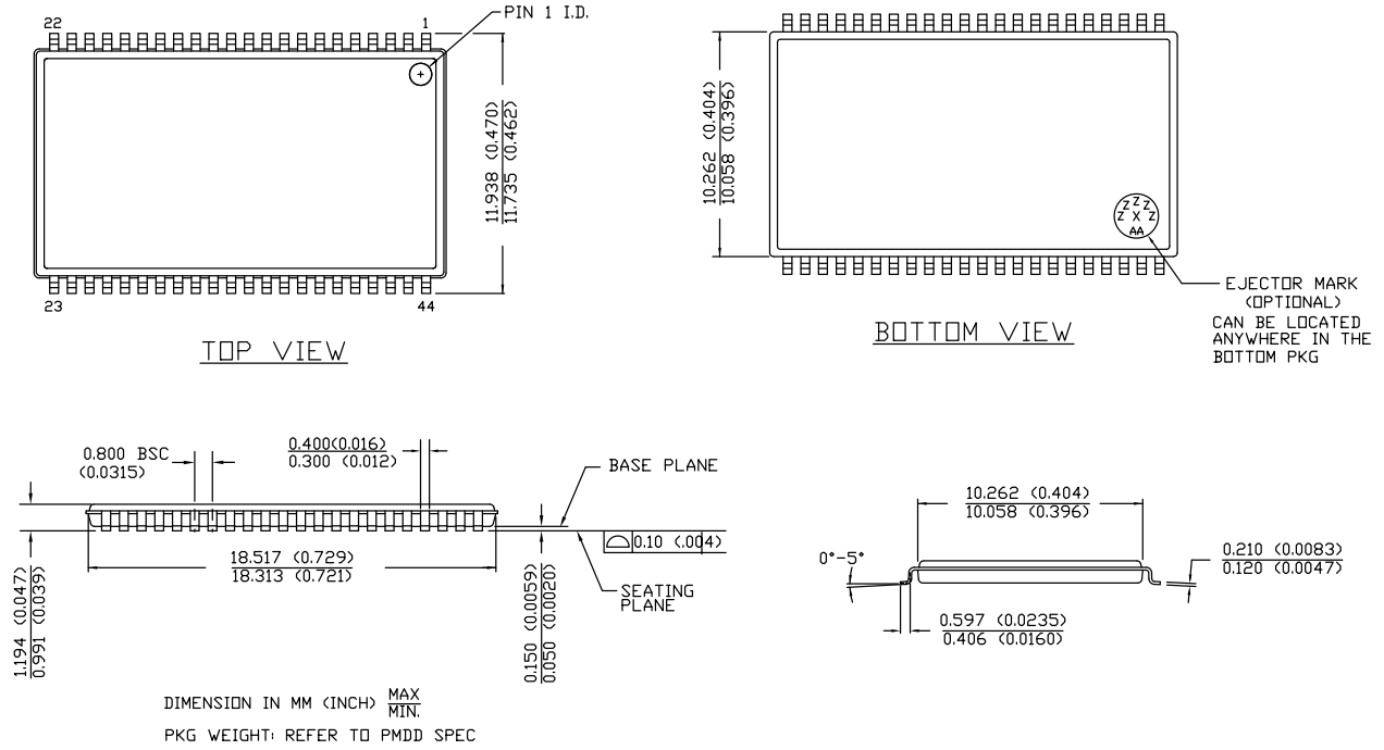
図 17. 44 ピン TSOP II パッケージ図、51-85087
