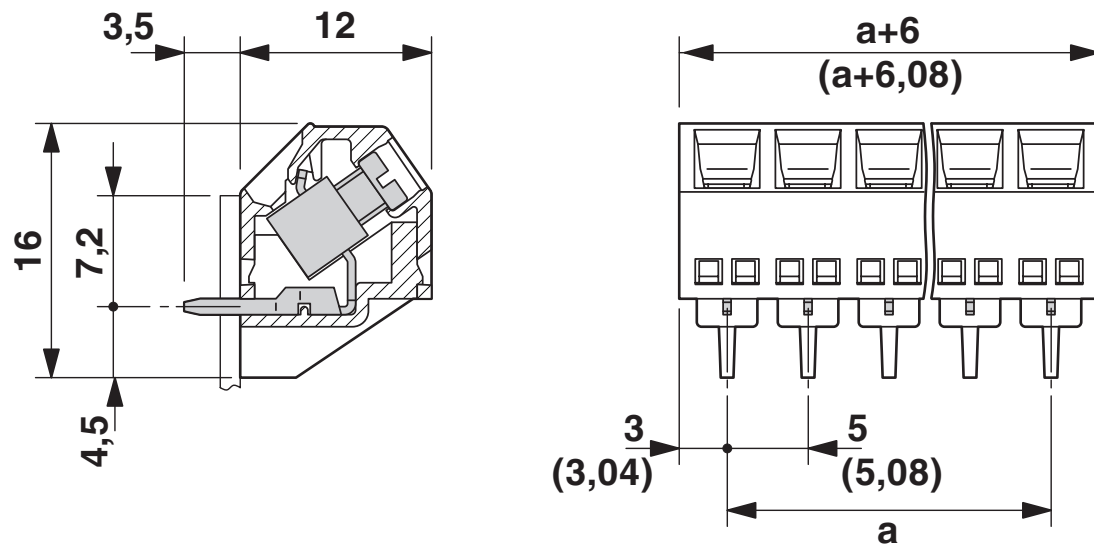
尺寸图
