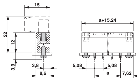
外形寸法
