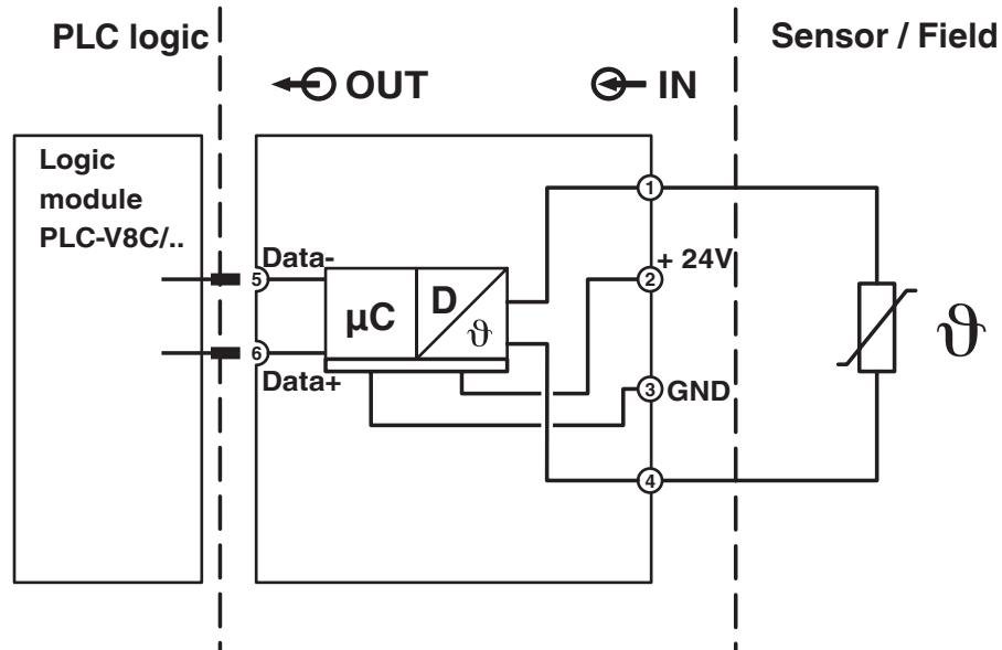
Blockschaltbild
