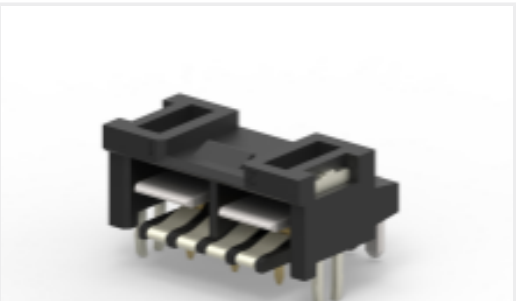
TE Part #1982295-1 ELCON MINI 2P RA HEADER, W /CODING
