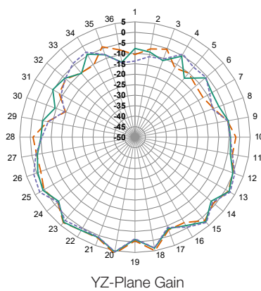
YZ-Plane Gain
