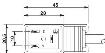
外形寸法
