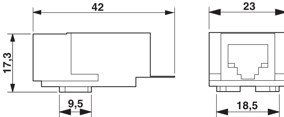
尺寸图
