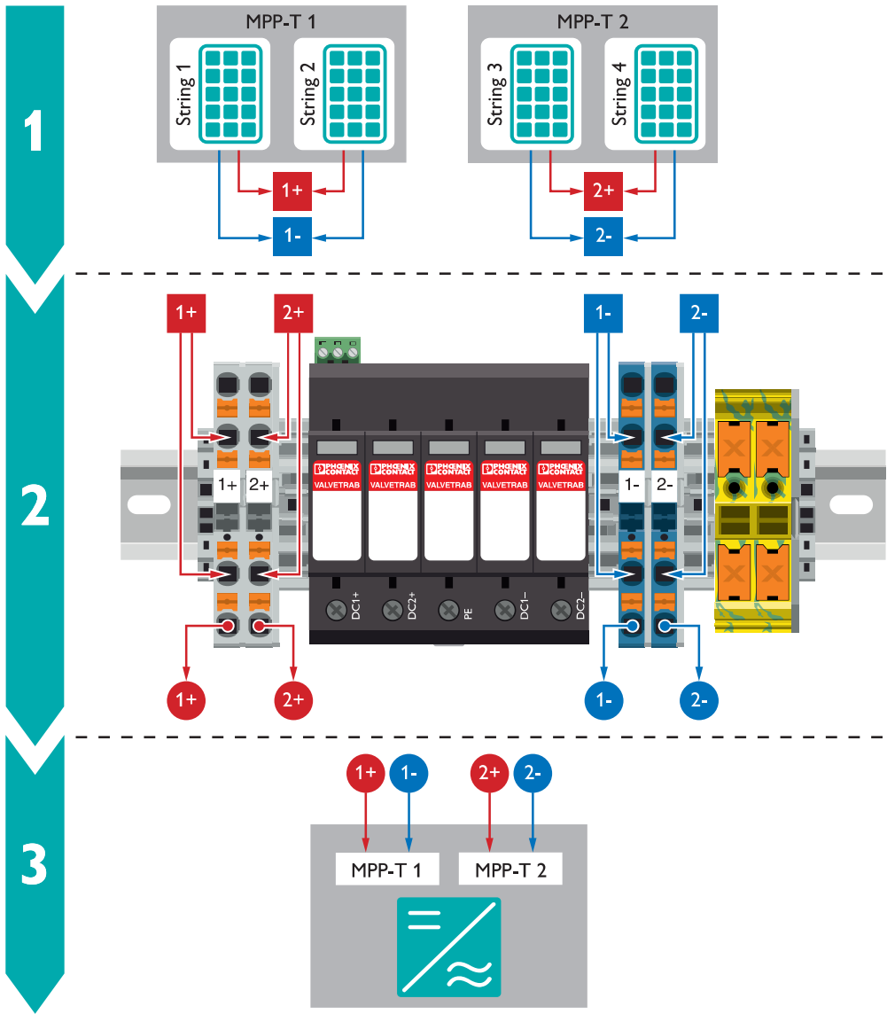
接线图
