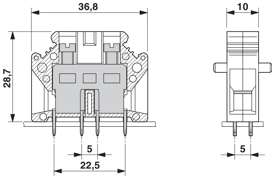
尺寸图
